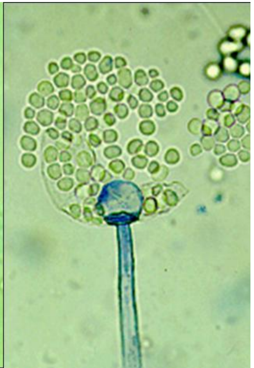
孢囊孢子 (Sporangiospore)
