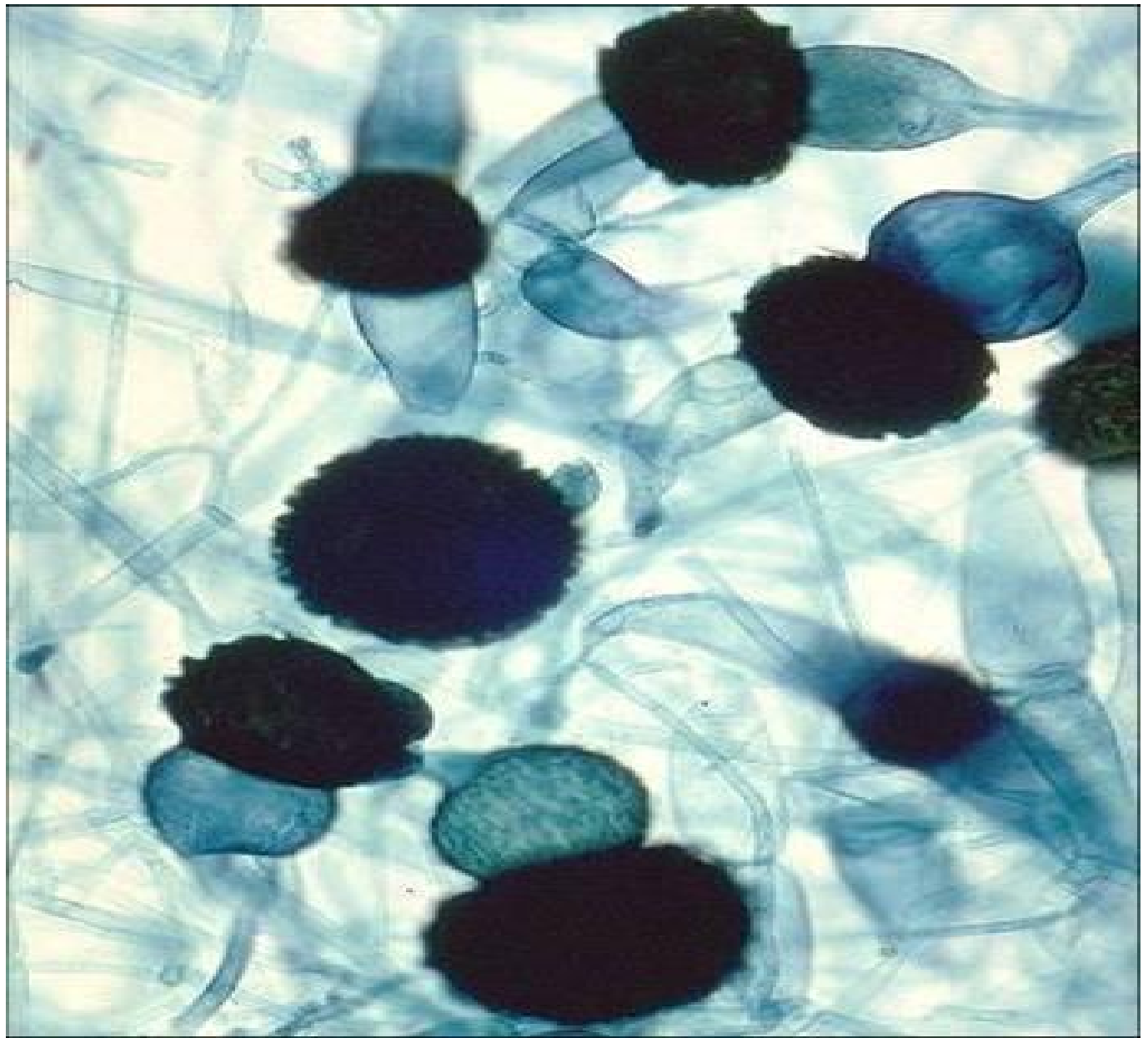
接合孢子 (Zygospore)
