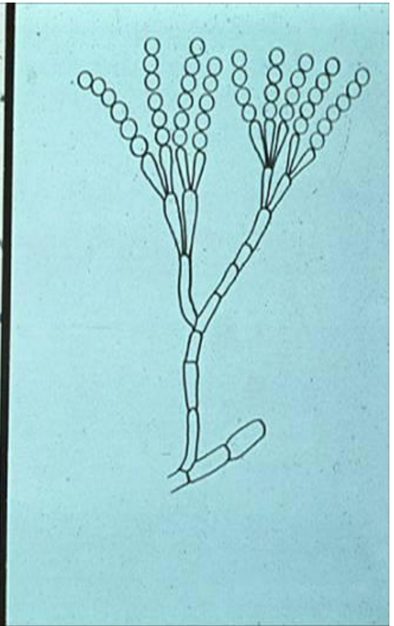
青霉的分生孢子头
