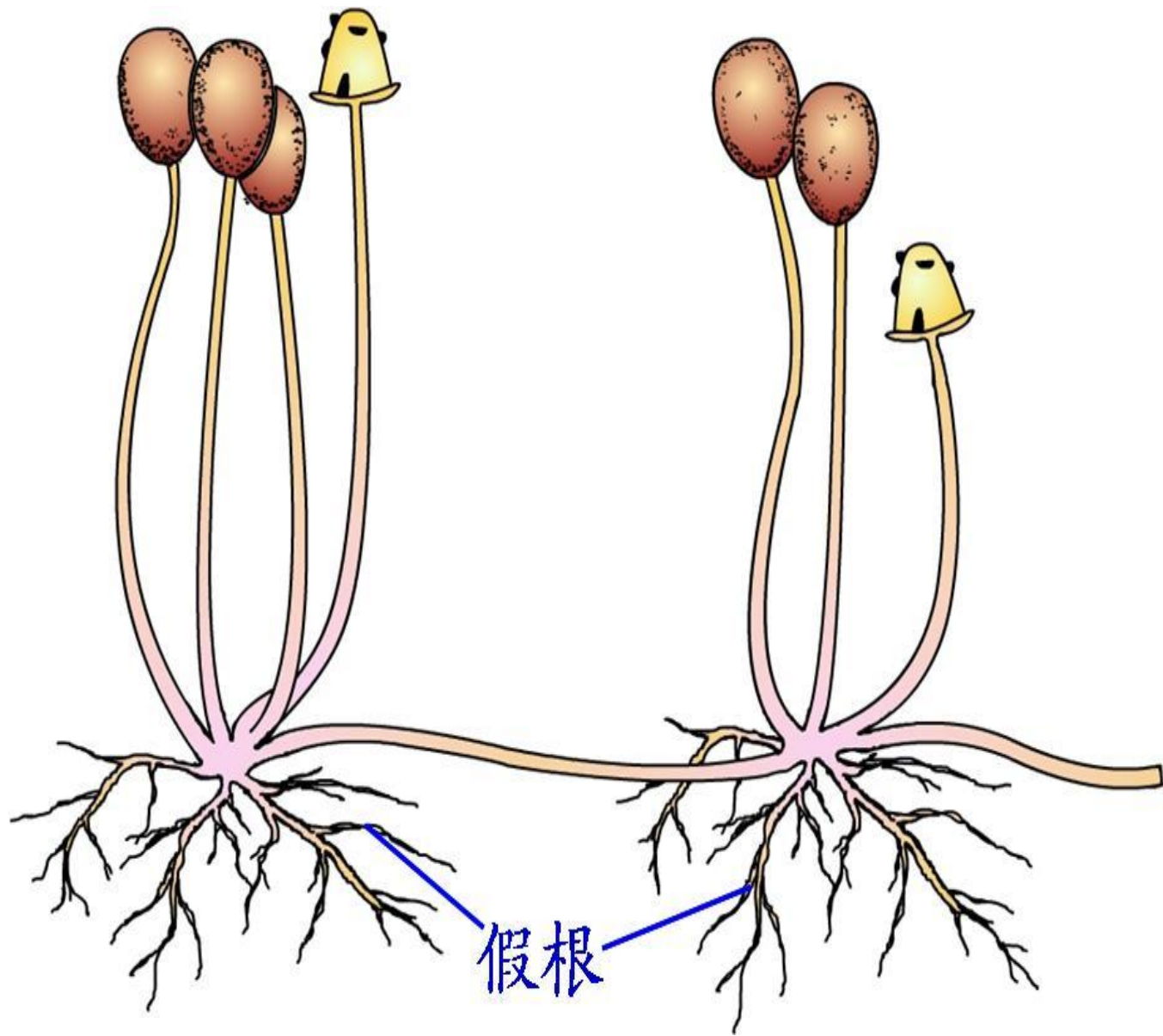
假根和孢子囊
